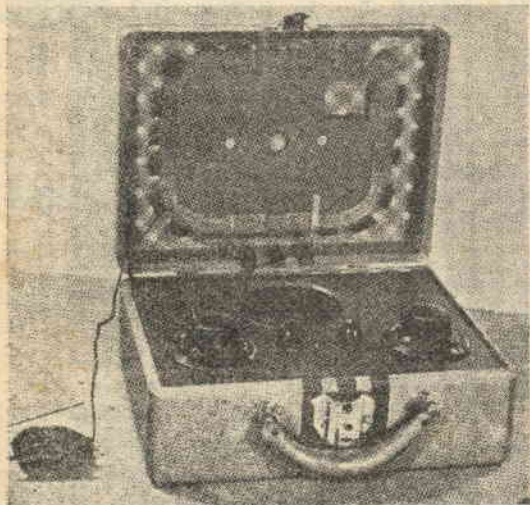
Fig. 4. - Come si presenta il ricevitore finito.
